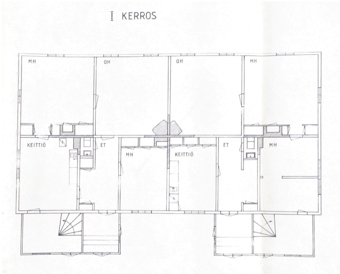
Kuva 25: Puukoulun ensimmäisen kerroksen pohjapiirros ennen 1980-luvun muutoksia. Piirroksessa näkyvillä vielä rakennuksen alkuperäinen huonejako pienin muutoksin. Kummasakin päädyssä on kolmen huoneen ja keittiön asunnot.
