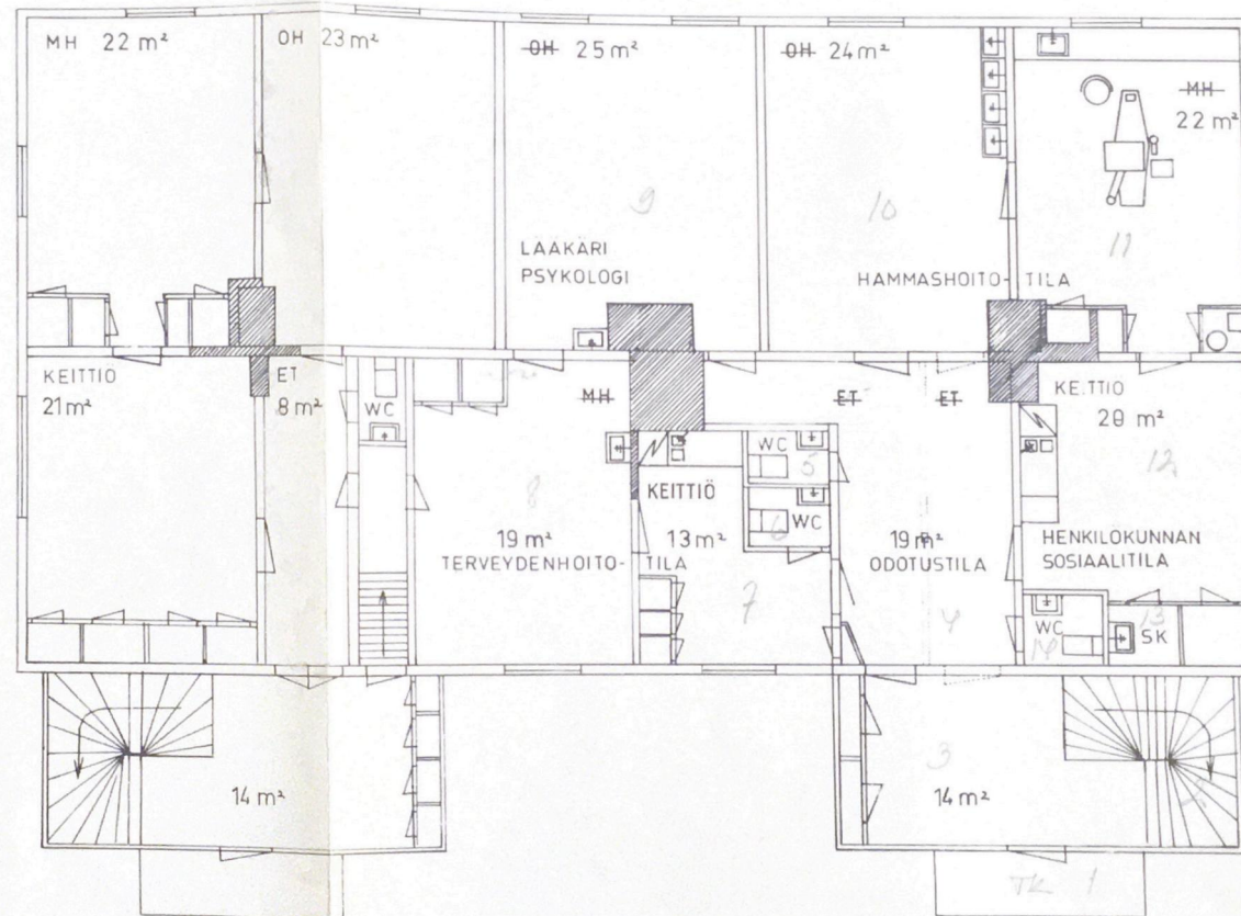
Kuva 26: Toisen kerroksen pohjapiirustuksessa näkyvillä alkuperäinen huonejako, jolloin siellä sijaitsi kolme asuntoa, joissa kussakin oli kaksi huonetta ja keittiö. Kun opettajilta vapautui asuntoja yläkerrasta, muutettiin ne terveydenhoitotiloiksi ja henkilökunnan sosiaalitiloiksi.
