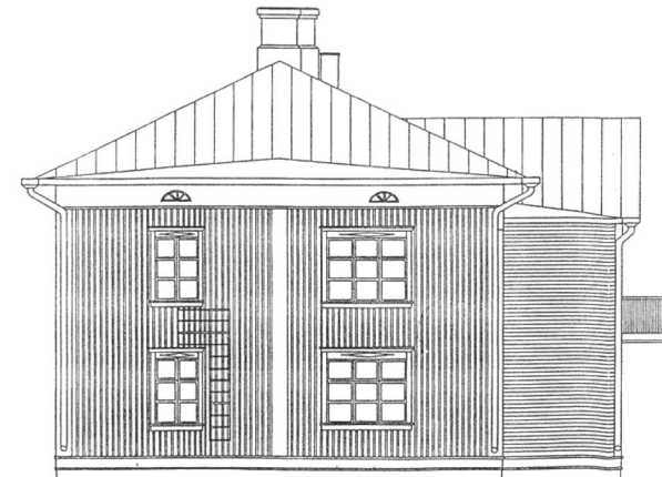
Kuvat 16-19: Nurkkakivi Ry:n dokumenttipiirustukset koulurakennuksesta. Vasemmalla ylhäällä eteläjulkisivu, joka näkyy koulukadulle. Vasemmalla alhaalla pohjoisjulkisivu, joka näkyy koulupihalle. Oikealla ylhäällä länsipääty ja oikealla alhaalla itäpääty.
