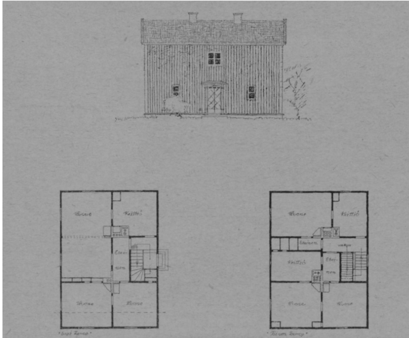
Kuva 12: Gunnar Taucherin suunnitelmat kaksinkertaisen yläkoulun ja alakoulun huoneistosta ja yläkoulun mies- ja naisopettajan sekä alakoulun opettajattaren asunnoista voittivat ensimmäisen sijan vuoden 1921 tyyppipiirustuskilpailussa. Kuvassa asuntolarakennuksen tyyppipiirustukset.
