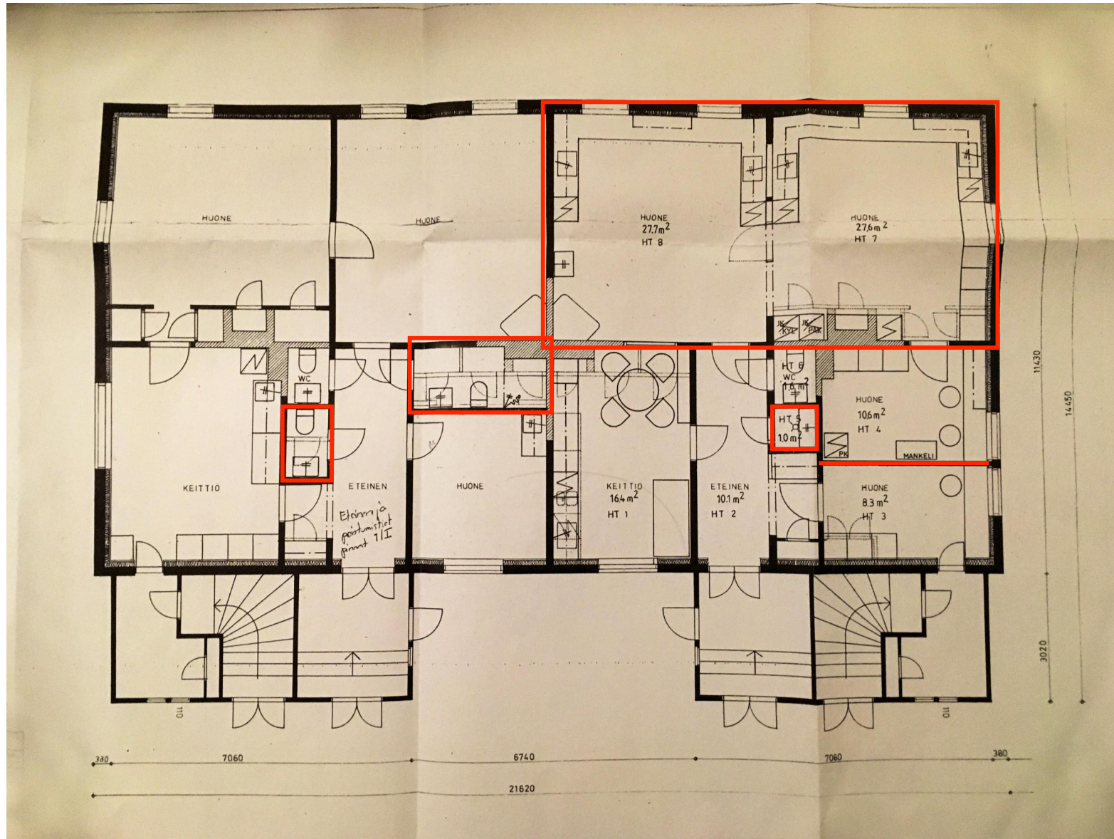
Kuva 27: Suunnittelupiirustus vuodelta 1982. Ensimmäisen kerroksen länsipään kaksi huonetta yhdistettiin harjaantumiskoulun opetuskeittiöksi. Länsipäädyn muissakin huoneissa tehtiin muutoksia (suurimmat muutokset korostettu kuvaan), mutta itäpääty jäi pääasiassa 1950-1960 -lukujen asuun.
