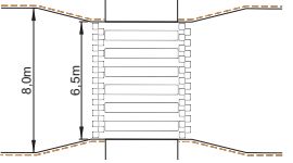
TASOKUVA 1:100 SUOJATIED KAVENNUS JA KOROTETTU SUOJATIE
