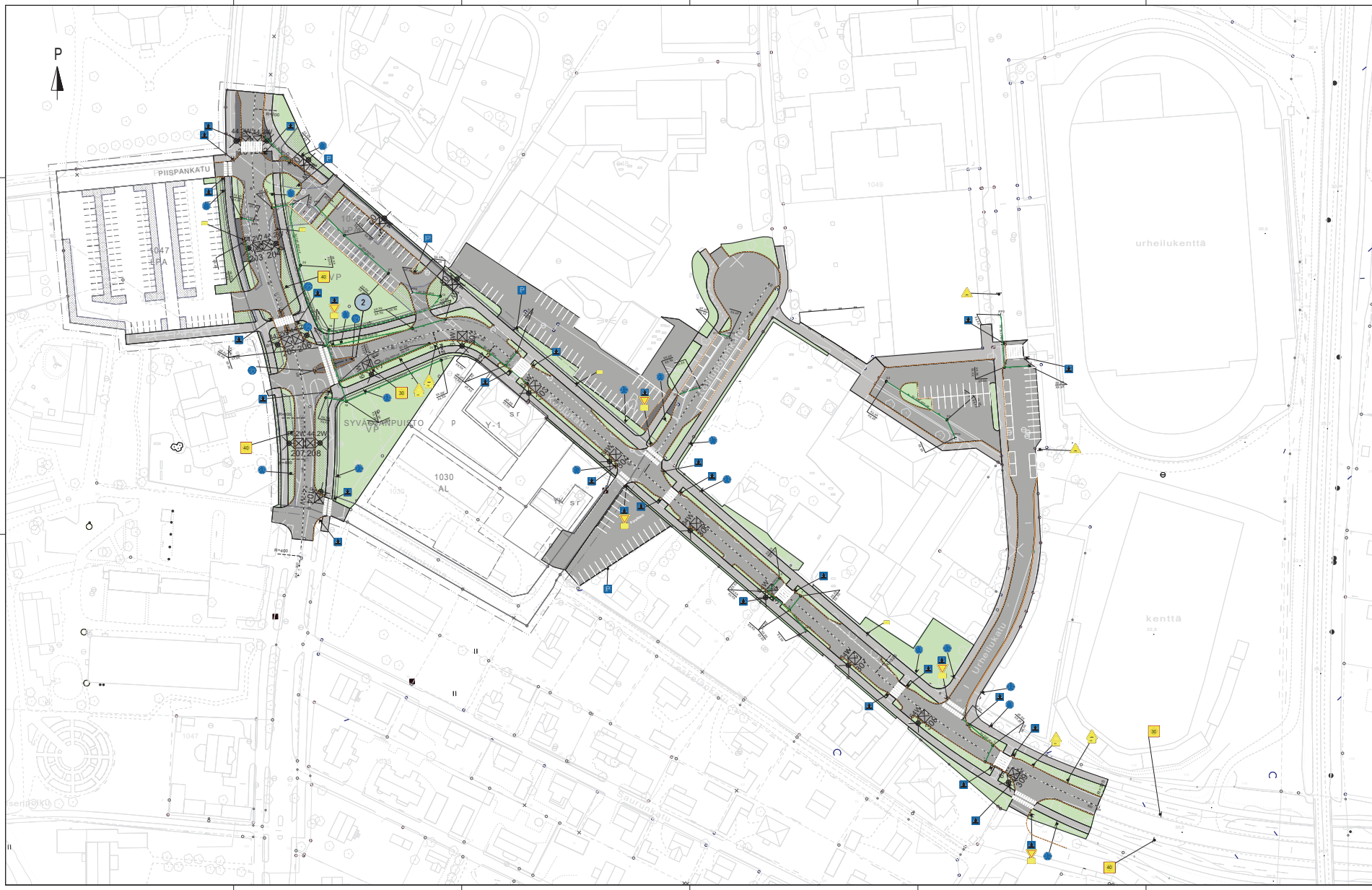
TASOKUVA 1:100 SUOJATIED KAVENNUS JA KOROTETTU SUOJATIE
